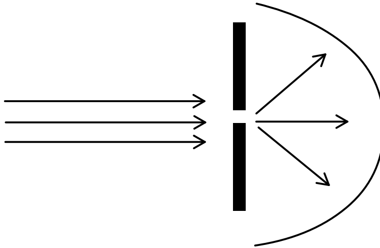
Abbildung 1: Gedankenexperiment von Einstein
