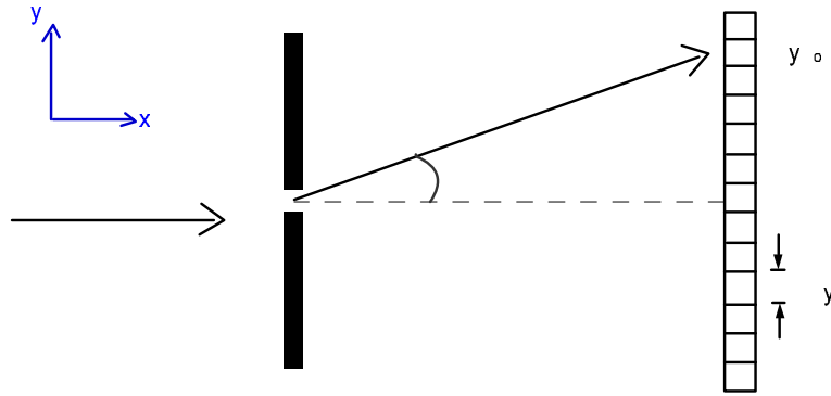
Abbildung 4: Gedankenexperiment zur Unbestimmtheitsrelation.
