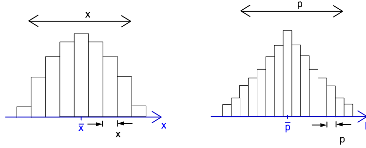
Abbildung 3: Meßfehler und Standardabweichungen für Ort und Impuls.
