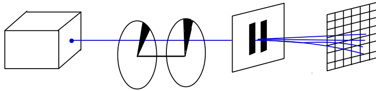
Abbildung 2: Versuchsanordnung zur Verdeutlichung von „Präparation“ und „Messung“.
